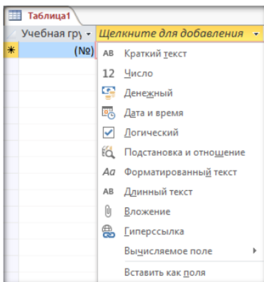
Рис. 3 – тип данных
