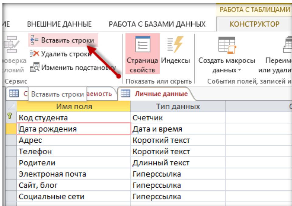
Рис. 23 – Добавление строк
