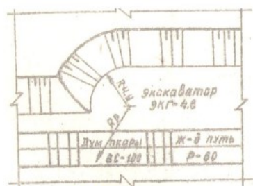
Рисунок 3. Упрощенное изображение механизмов на горных чертежах.
