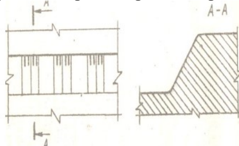
Рисунок 2. Изображение добычного уступа.
