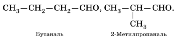
Бутаналь
