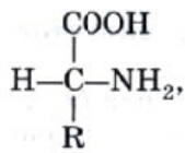
D-аминокислота
