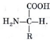
L-аминокислота
