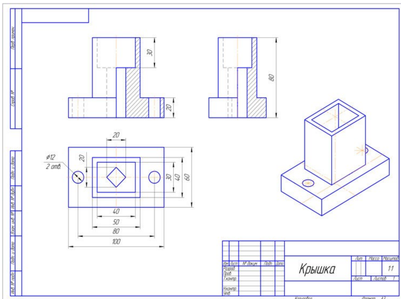
Рис. 3 Образец выполнения.
