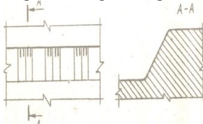
Рисунок 2. Изображение добычного уступа.
