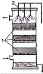
Орошаемая противопоточная насадочная башня
