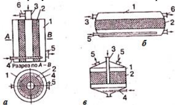
Конструктивные схемы адсорберов
