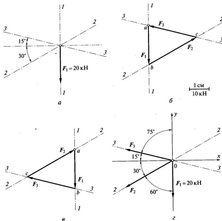
а — заданная схема действия сил; б, в — варианты построения силового треугольника; г — схема сил для аналитического решения
