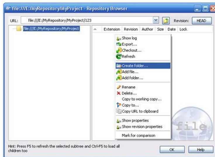
Рис.1.5 Обзорщик хранилища
