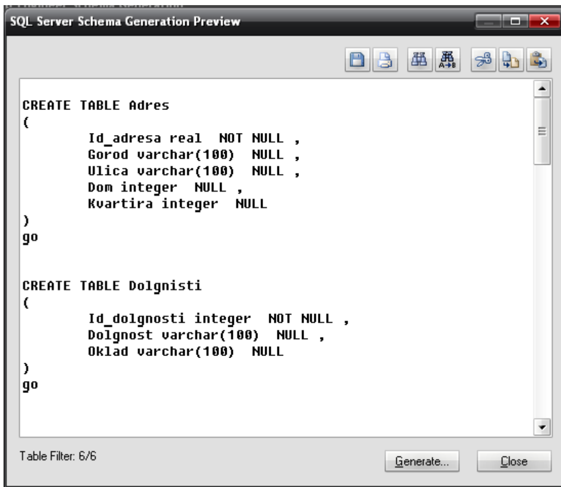
Рис.10. Генерация SQL-кода для MS SQL
