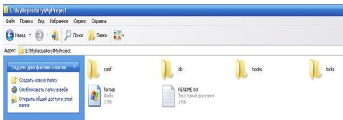
Рис.1.4 Структура репозитория
