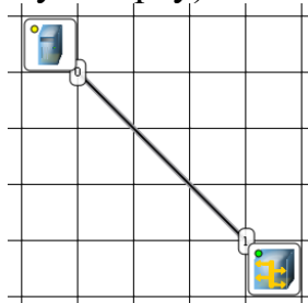
Добавляем интерфейс
