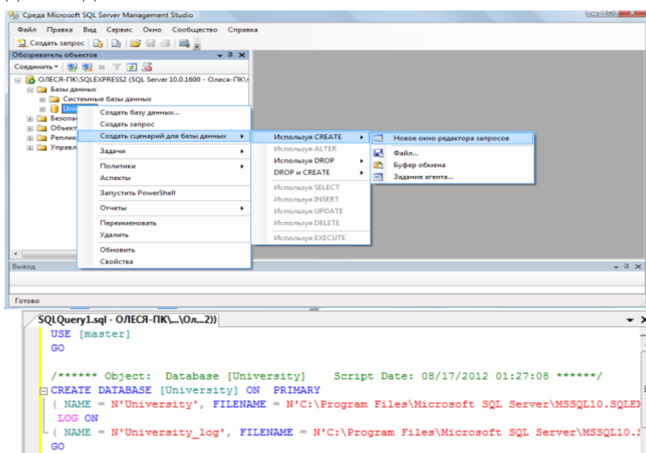
Рис. 2. Сгенерированный sql-код созданной базы данных
