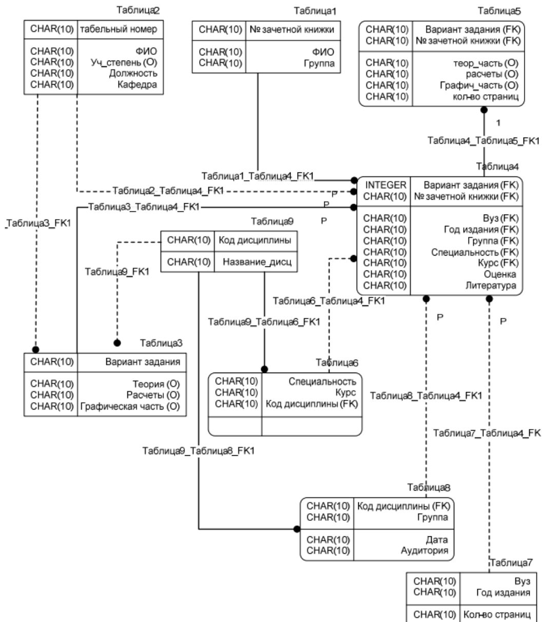
Рисунок 17 – Вид физической модели
