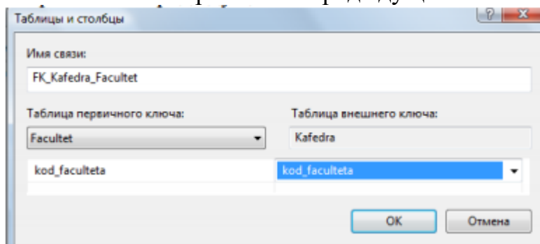
Рис. 7. Создание Внешних ключей
