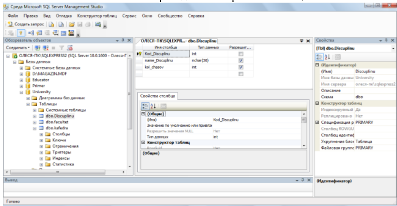
Рис. 2. Окно формирования таблицы в диалоговом режиме Сетка в средней части окна содержит сведения о полях таблицы.
