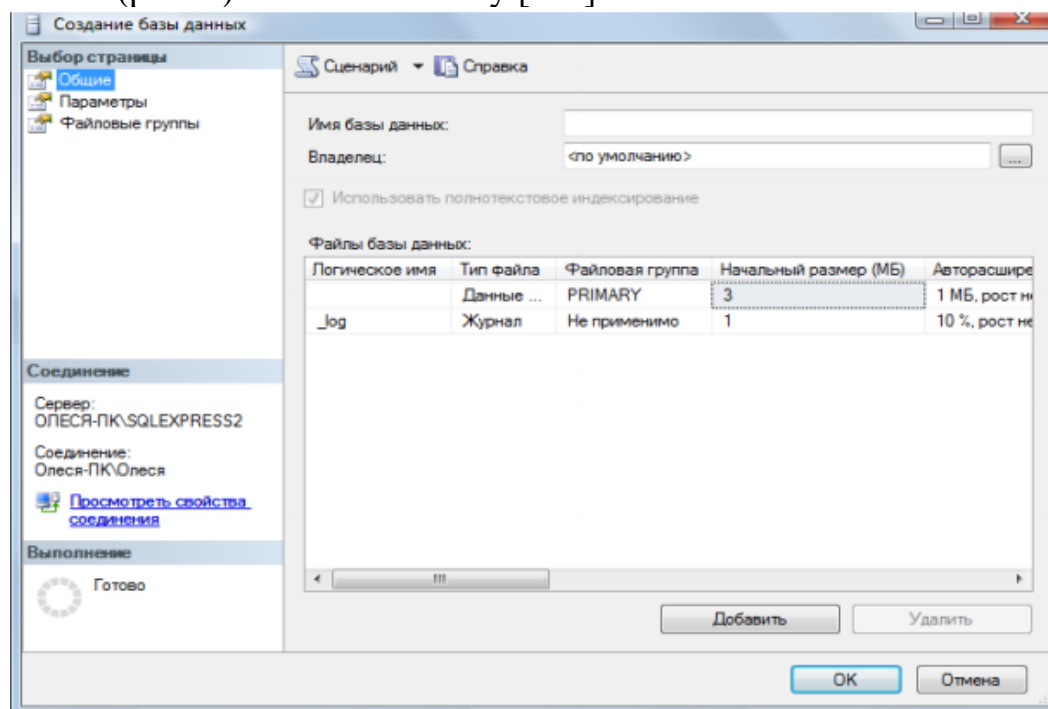
Рис. 1. Диалоговое окно создания базы данных
