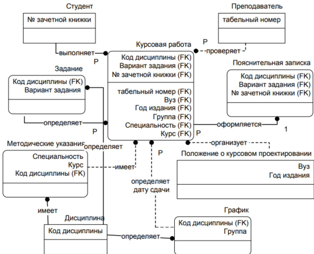
Рисунок 11. – Скорректированная информационная модель, основанная на ключах.
