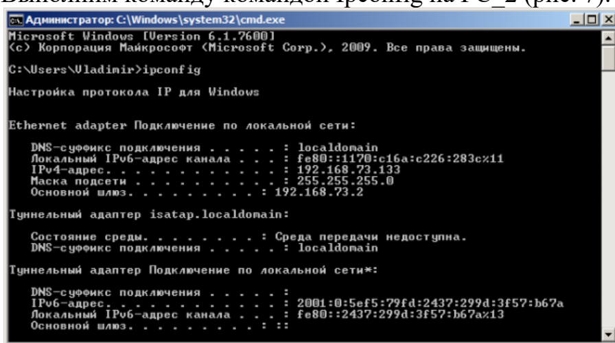
Рис. 7 Отображение параметров TCP/IP-протокола командой Ipconfig
