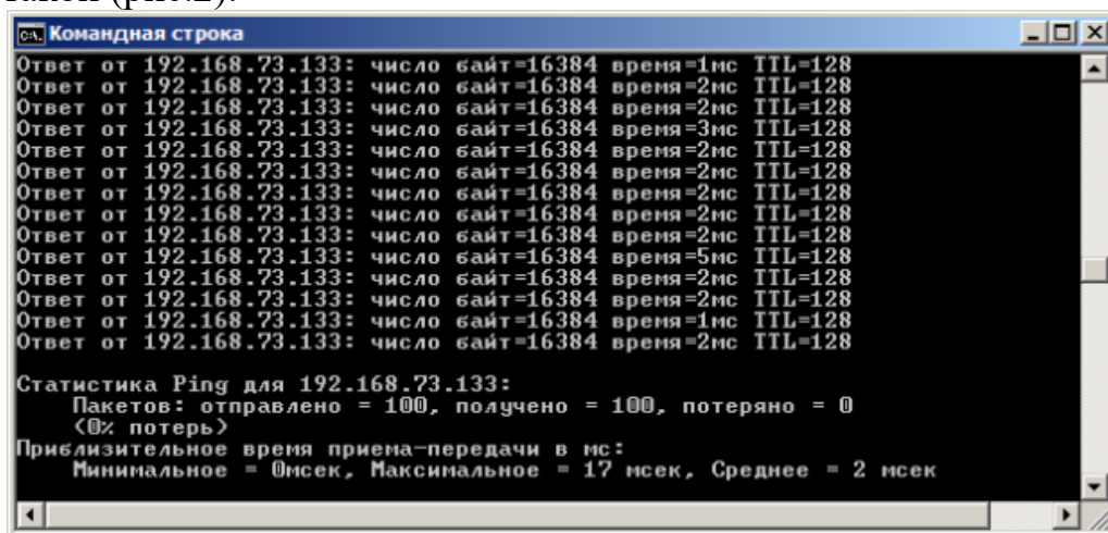
Рис. 2 Ответ на команду ping.exe с ключами
