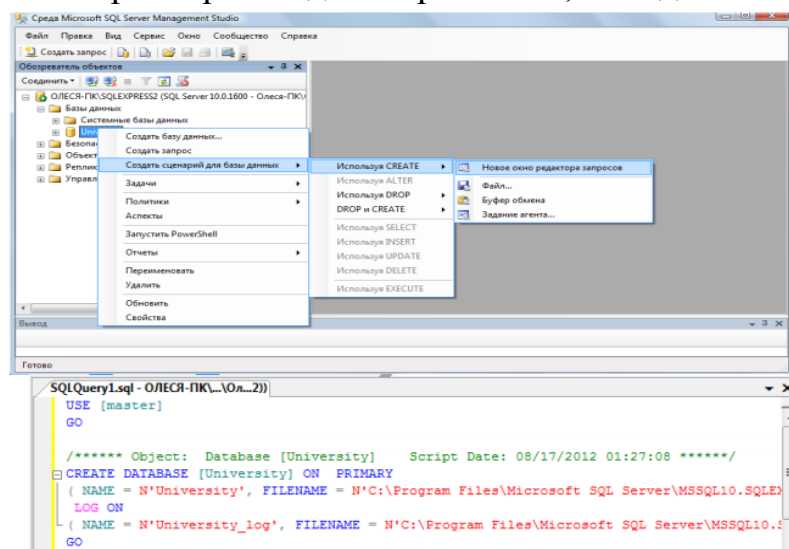
Рис. 2. Сгенерированный sql-код созданной базы данных
