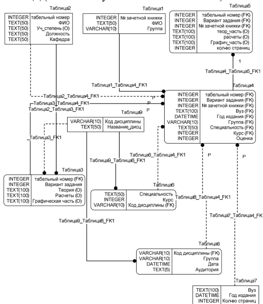
Рисунок 19 – Физическая модель базы данных
