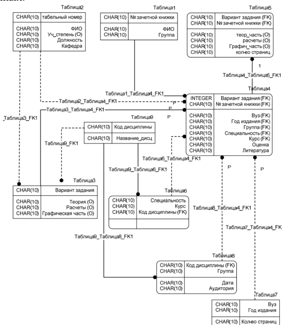
Рисунок 17 – Вид физической модели
