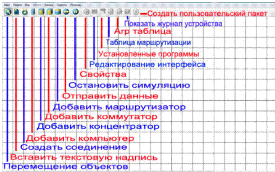
Интерфейс программы Netemul
