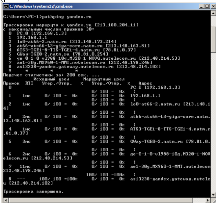
Рис. 5. Пример использования утилиты Pathping Проанализируем результат:
