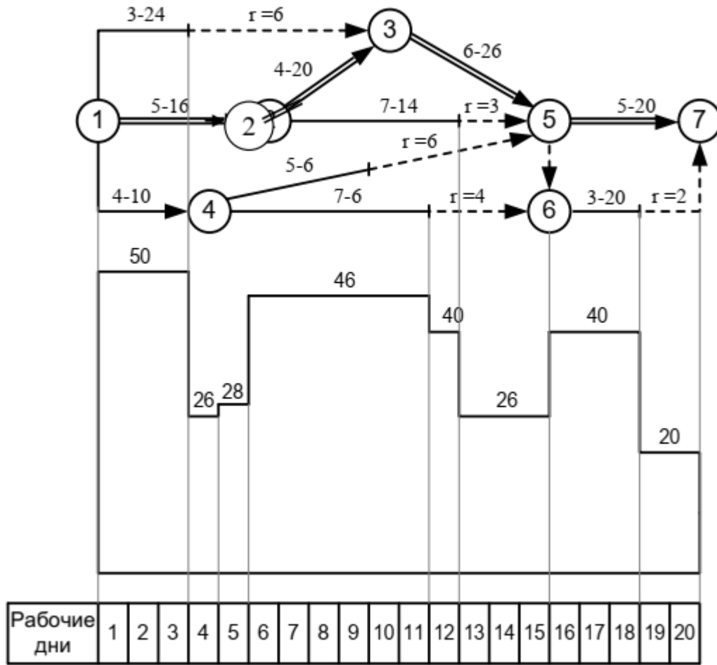
Сетевой график и график потребности рабочих после оптимизации
