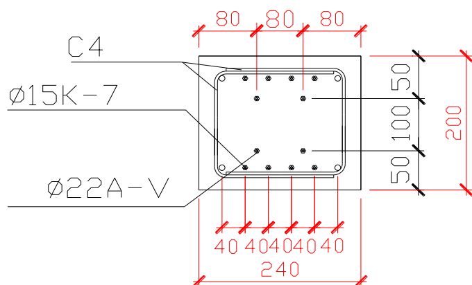
Рисунок 9. сечение нижнего пояса
