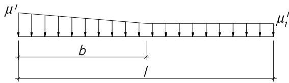
Рисунок 2. Схема распределения снеговой нагрузки на участке у перепада высот
