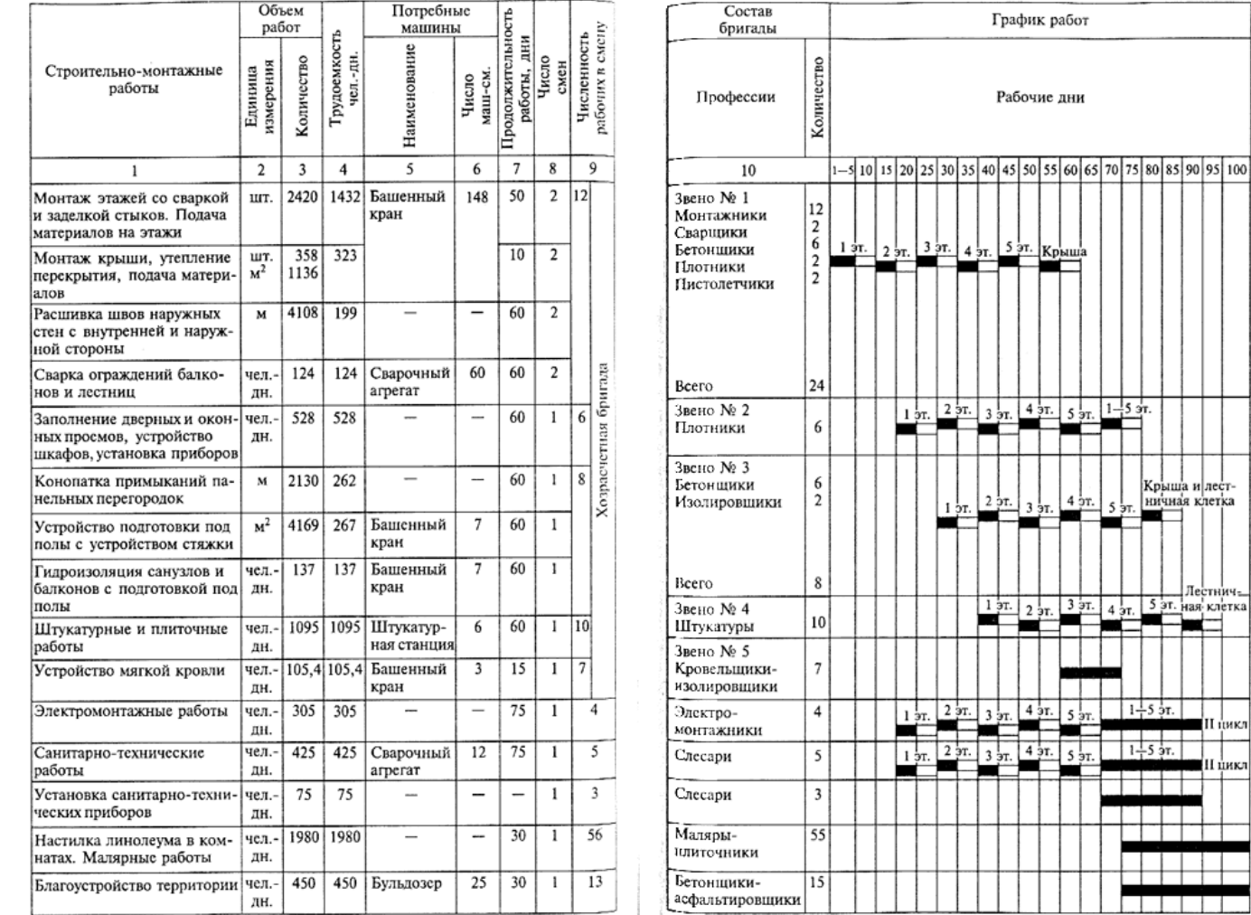
Рис.2. Календарный план производства работ по возведению кирпичного жилого дома При составлении календарных графиков выделяют выходные и праздничные дни. Это выделение производится при привязке разработанного графика к конкретной дате начала строительства. Итог работы: Отчет оформляется на листах формата А4 в соответствии со структурой: титульный лист, исходные данные, график. Практическая работа № 10. Цель: научиться составлять графики движения рабочих.
