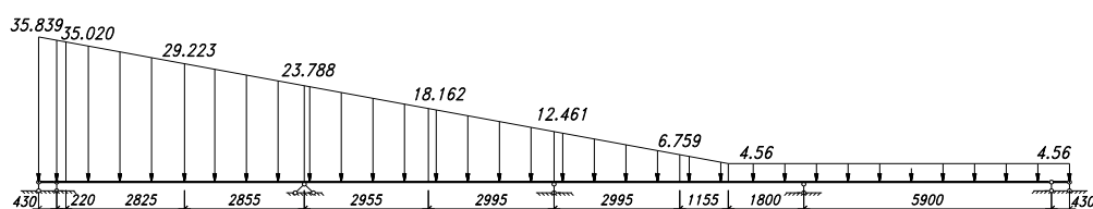
Рисунок 7. Схема третьего варианта загрузки снеговой нагрузкой
