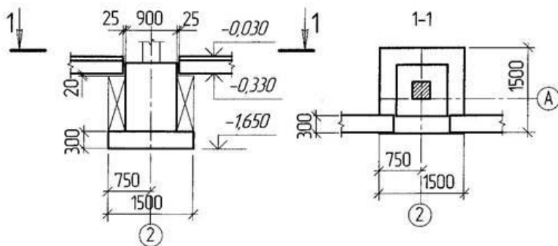
Узел опирания фундаментной балки на фундамент
