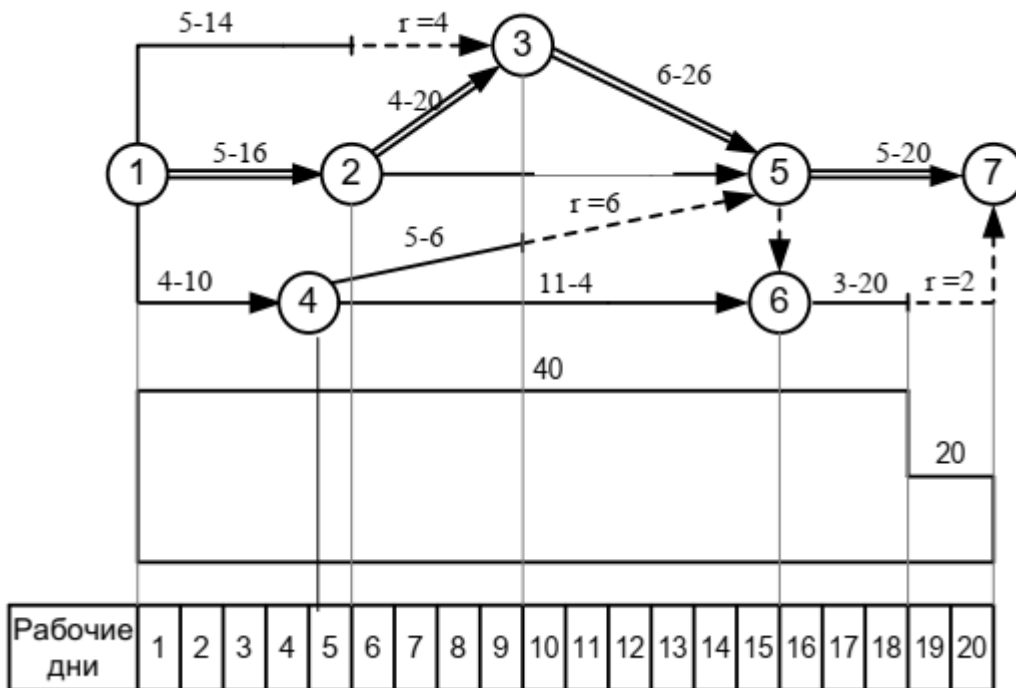
Сетевой график и график потребности рабочих после оптимизации
