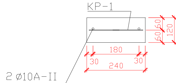
Рисунок 12. Сечение первого раскоса
