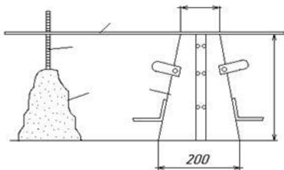
Рисунок 16. определение подвижности бетонной смеси стандартным конусом.
