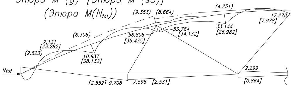
Рисунок 8. Эпюры M кНм
