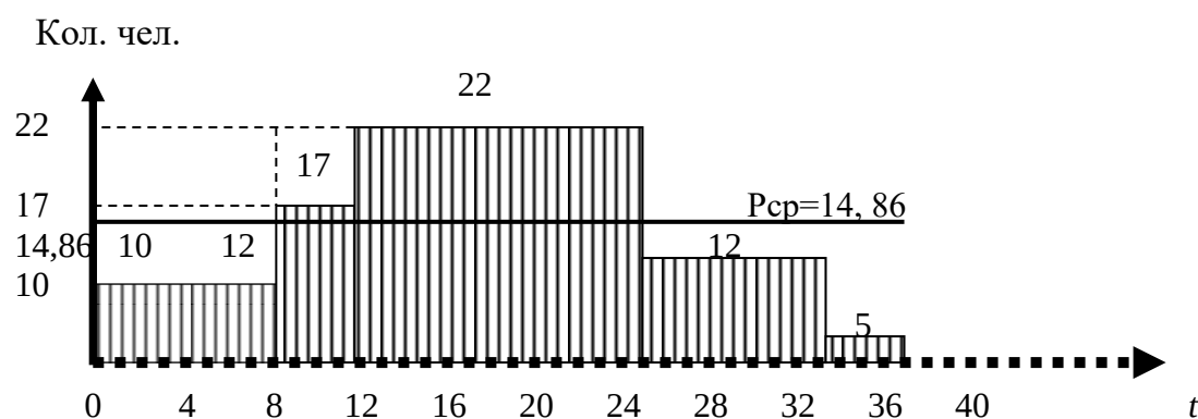
Рис. 33. График движения рабочей силы
