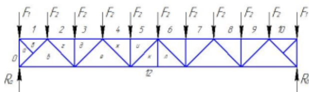
Схема фермы
