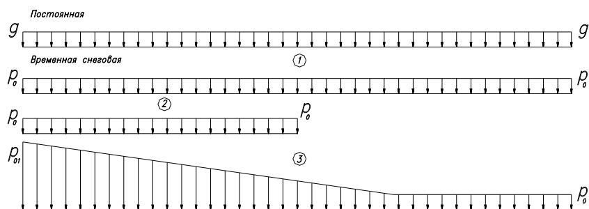
Рисунок 6. Геометрическая схема и схема передачи нагрузки на ферму
