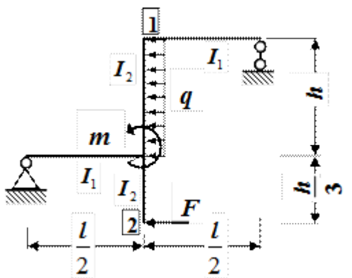
Рис.25. Схема рамы
