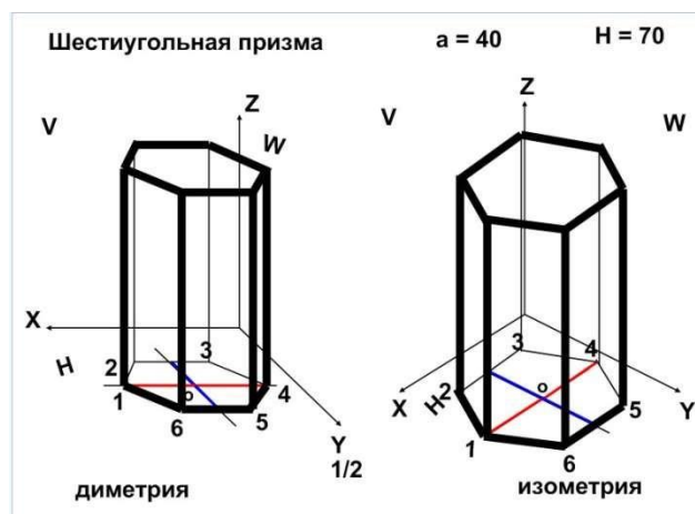
Рисунок 11.1-Пример выполнения задания
