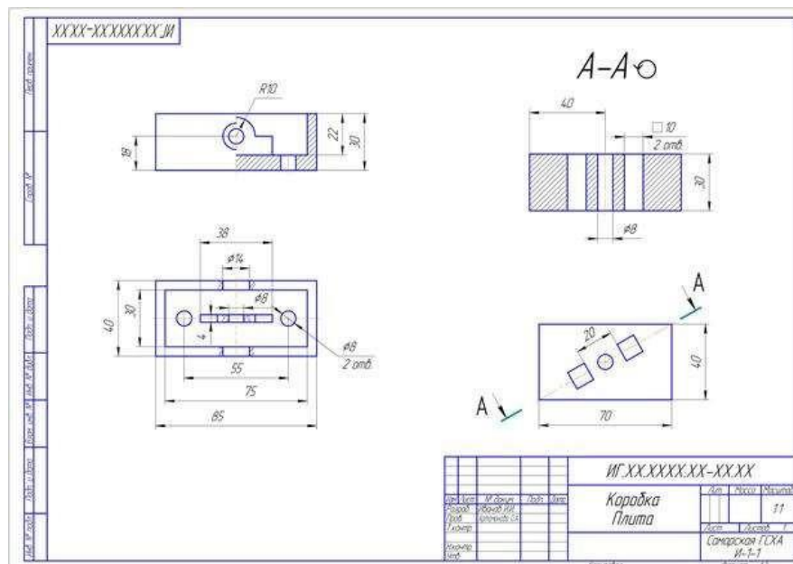
Рисунок 25.1- Пример соединения части вида с частью соответствующего разреза, построения наклонного разреза с поворотом его изображения. Итог работы: Студент сдает практическую работу преподавателю в установленный срок, отвечая на контрольные вопросы к чертежу, поясняя ход выполнения практической работы.
