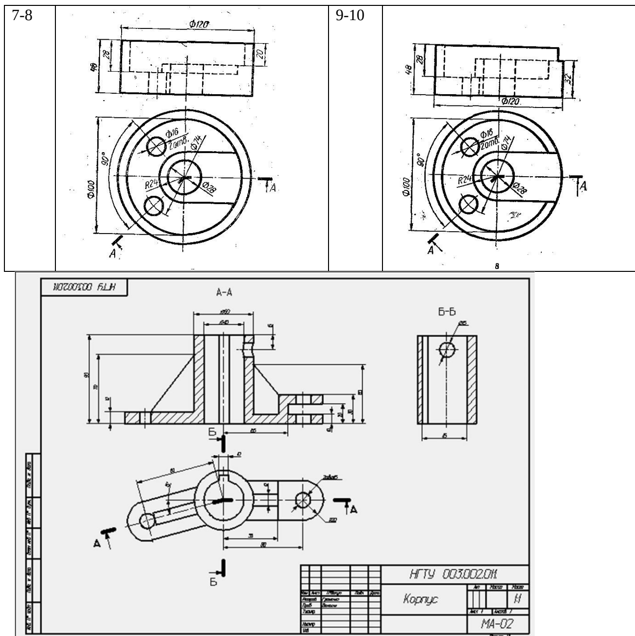
Рисунок 27.1-Пример выполнения ломаного разреза
